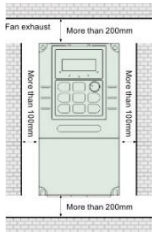
شکل 2-6 فضا و فاصله نصب
