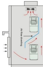
شکل 1-6 نصب چند اینورتر
