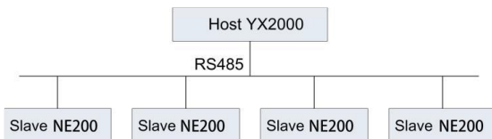
شکل 2-12 نمودار شماتیک شبکه ارتباطی چند ماشینه
