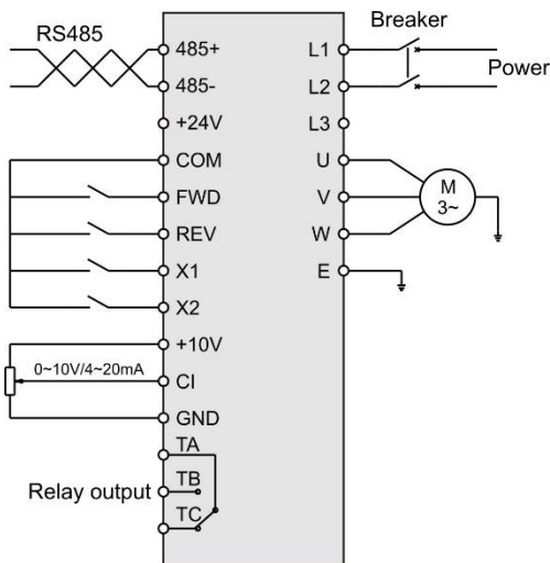
شکل 8-1 نمودار سیم بندی اولیه
