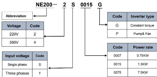
شکل 1-2 توضیح مدل اینورتر
