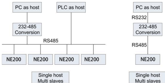
شکل 1-12 نمودار شماتیک شبکه واحد
